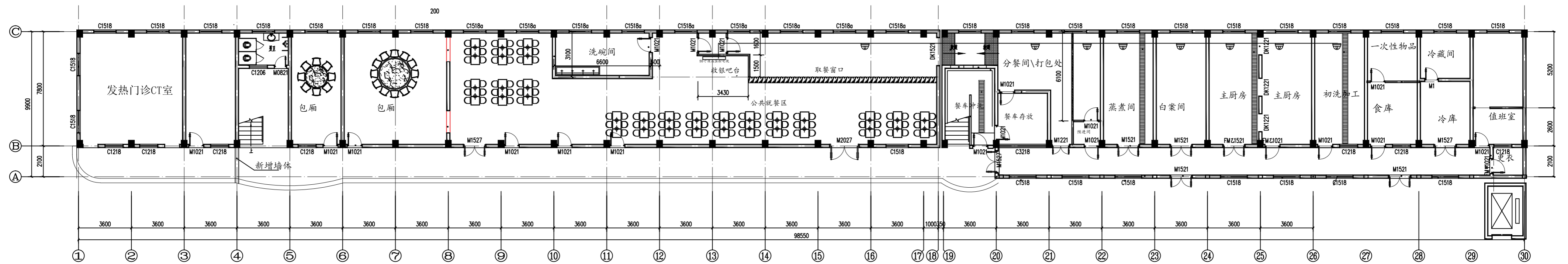
一层平面图 1:100
